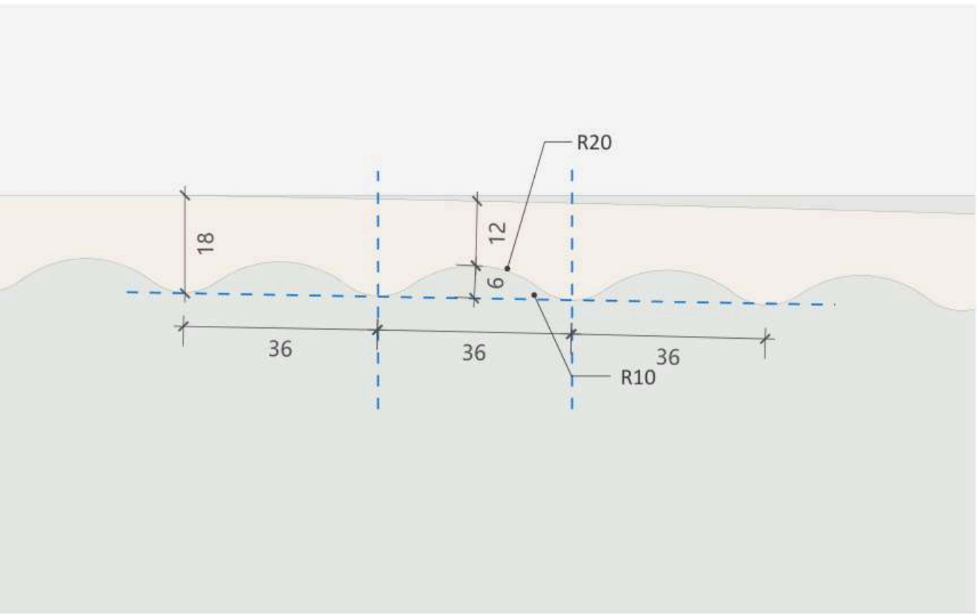
GRG造型深化
