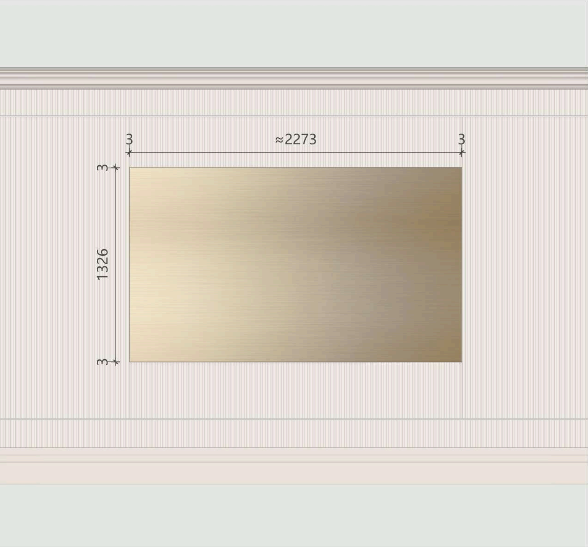
金属框与上下GRG关系：金属框外凸3mm
